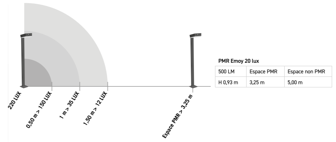
IMPLANTATION LUX /DISTANCE TEST RÉALISÉ AVEC UNE BORNE TD07K106 500 LM
